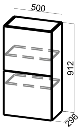
Ш5006(Aventos HF)
