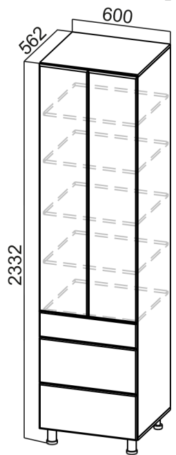
П600яг (600x2332x562)
