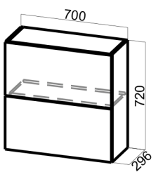
Ш700б(Aventos HF)
