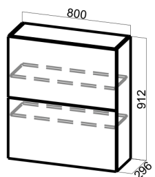
Ш8006(Aventos HF)
