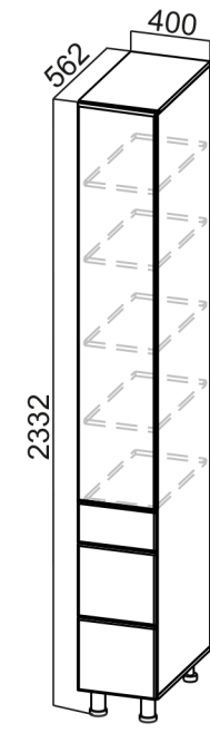
П400яг (400x2332x562)
