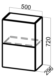
Ш500б(Aventos HF)
