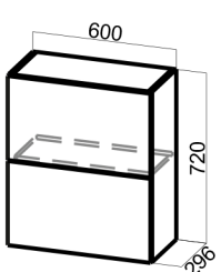
Ш600б(Aventos HF)
