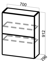
Ш7006(Aventos HF)
