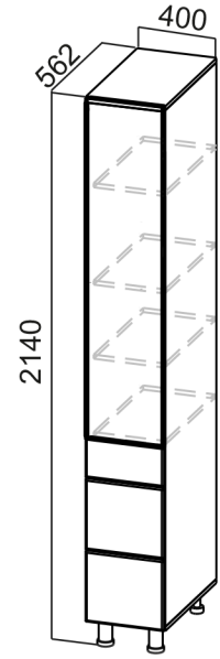
П400яг (400x2140x562)
