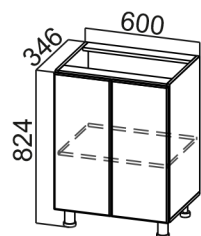
C600(400)*** 1. 600x824x346 2. 600x850x400
