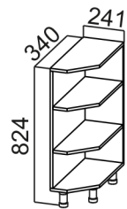
C300то(400)*** 1. 241x824x340 2. 300x850x400
